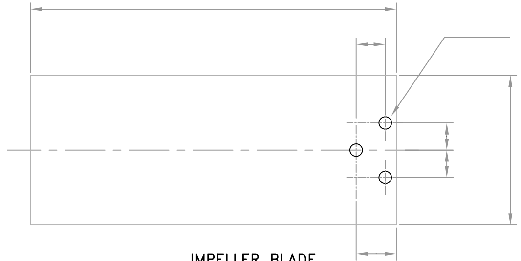
IMPELLER BLADE (4-OFF PER IMPELLER)
